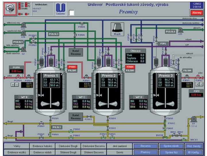
Obr. 2 Vizualizace části řízené technologie systémem Woderware Intouch
