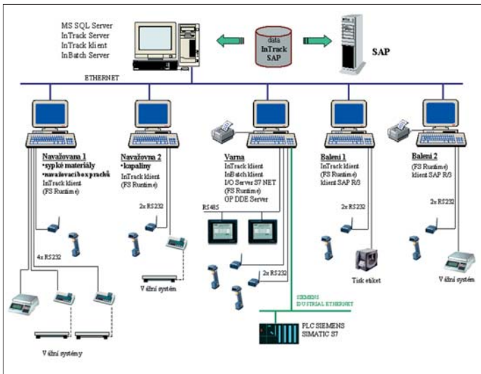
Obr. 1 Topologie systému pro řízení výroby v PTZ Nelahozeves
